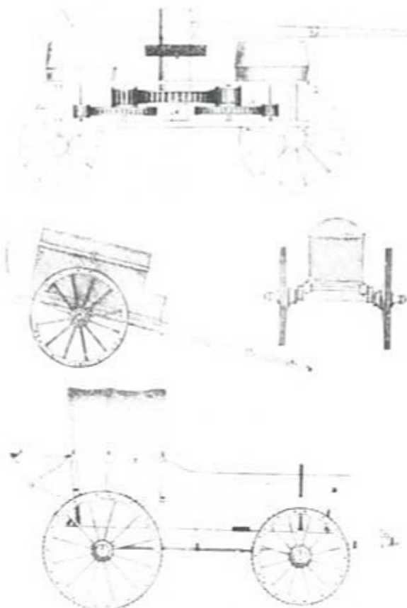
Svenska trängfordon på 1700-talet. Kvarnvagn från Karl XII:s tid. Brödkärta. Packvagn. Modellritningar i Krigsarkivet.
